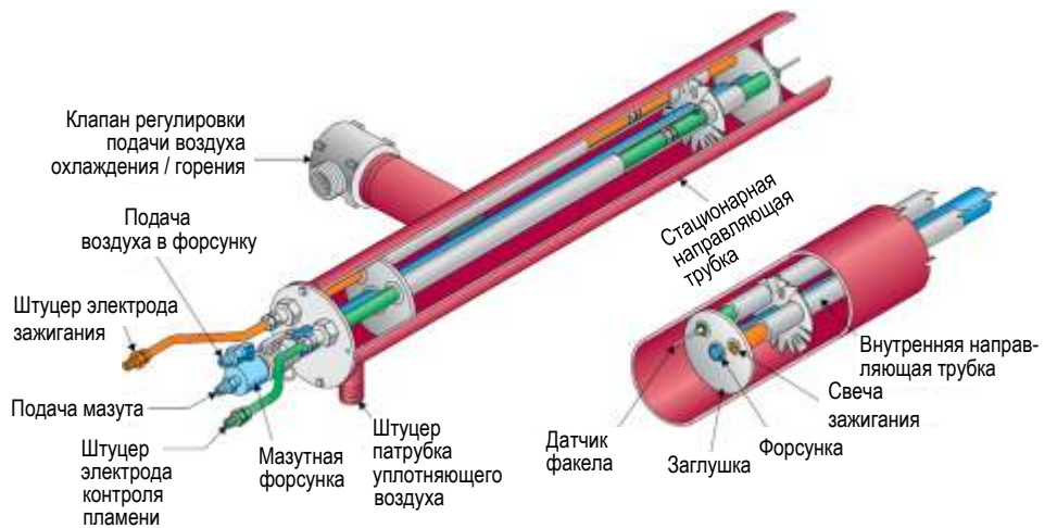
Мазутный запальник
