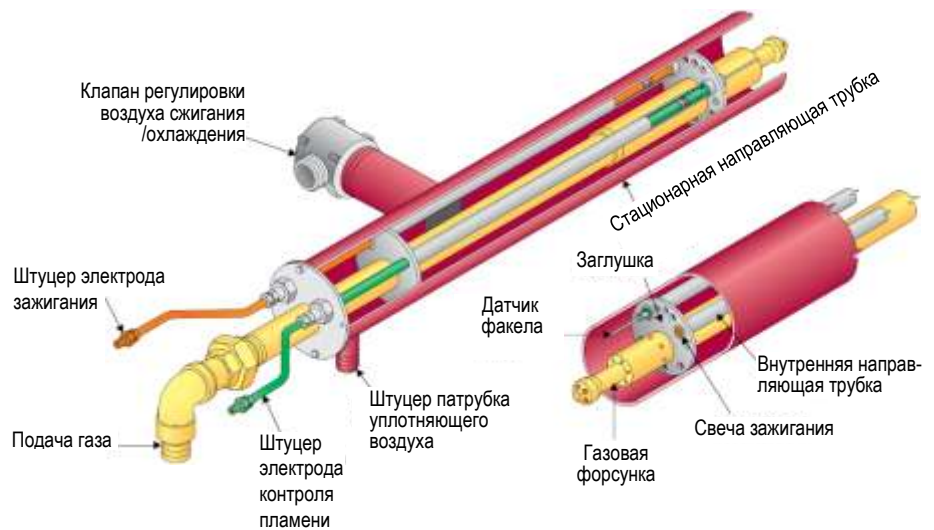
Газовый запальник
